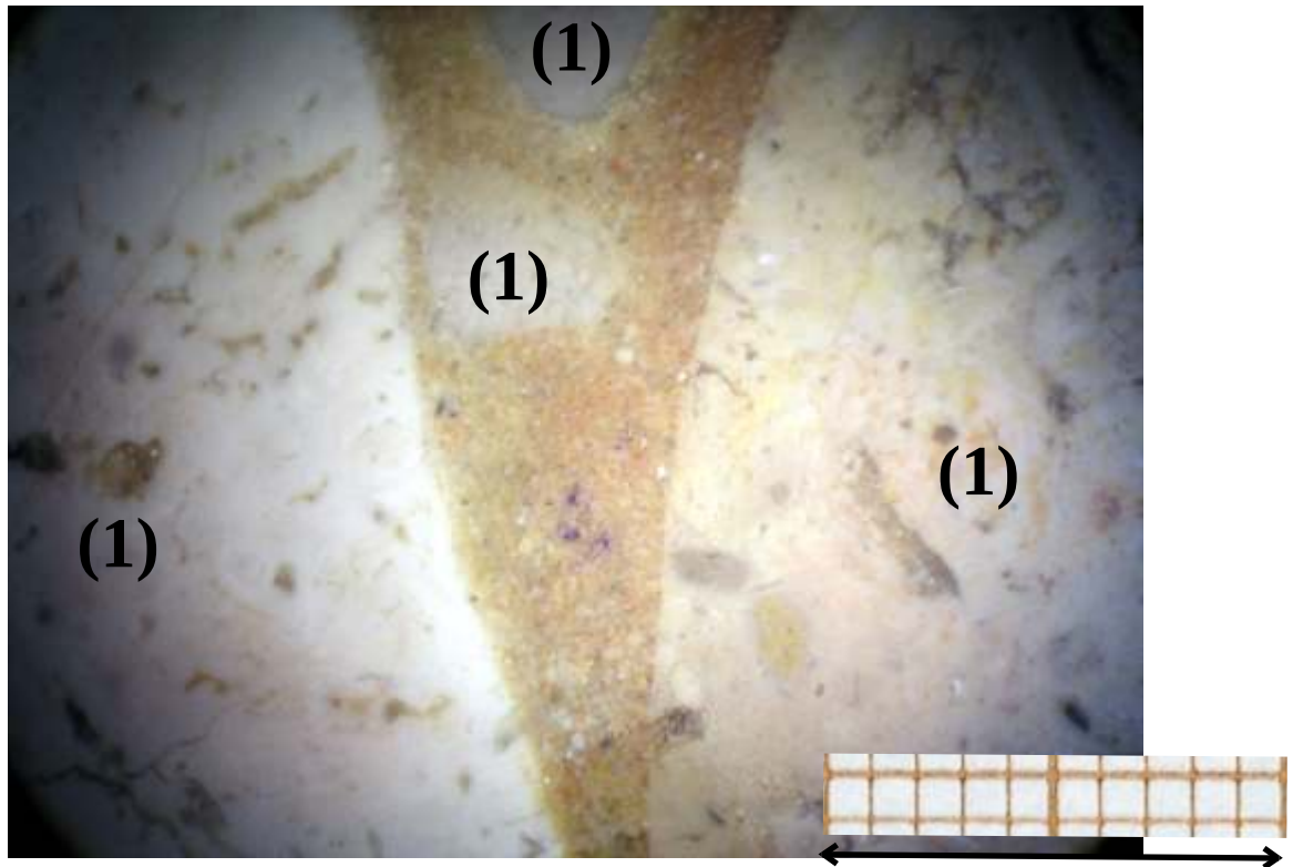
02_2 : Conglomérat à éléments et ciment carbonatés. 1 cm
